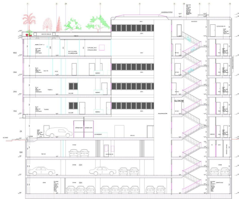
BB KESİTİ Ö=1/50
